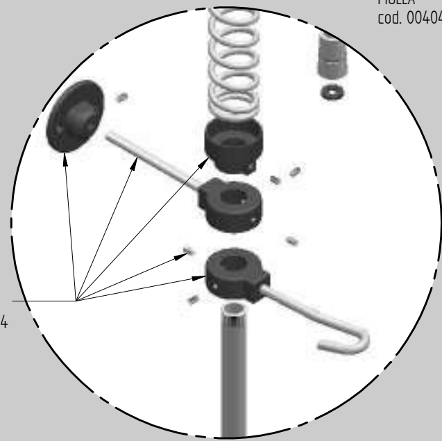
DETTAGLIO A
